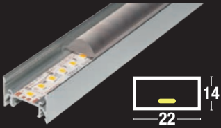
smartLED L1422 15°, 30°, 60°- und Asym-Optik
