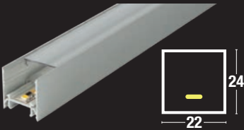
smartLED L2422 15°- und 30°-Optik
